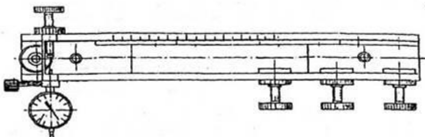
Рис. 8. Устройство для испытаний клинкового холодного оружия на прочность и упругость.
